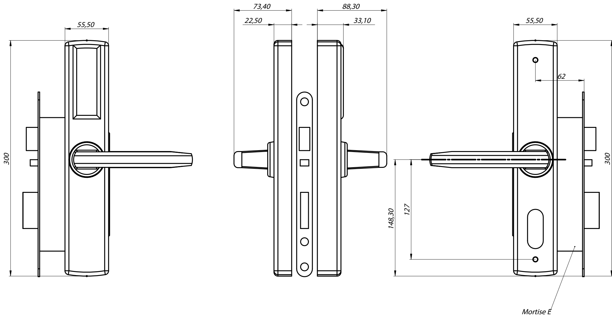
Rysunek złożeniowy szyldu elektronicznego LOB 5500 Adel z dedykowanym zamkiem wpuszczanym E
